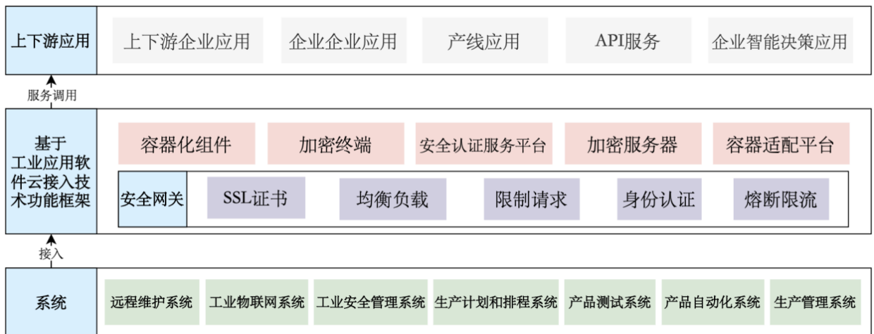
图 1 工业应用软件安全云接入功能框架
